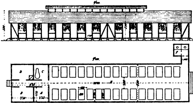
Č. 446. a 447. Baráková nemocnice.
